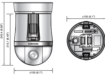
SCP-3370
